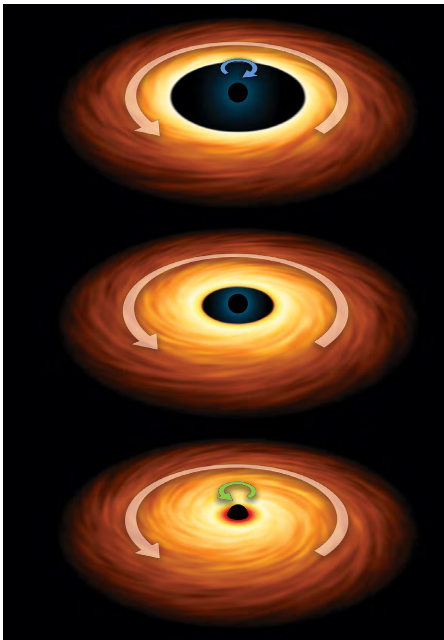
Na směr rotace černé díry závisí vzdálenost akrečního disku od horizontu událostí. Pokud černá díra rotuje v opačném směru než akreční disk, vzdálenost je větší než v případě, že se otáčí ve stejném směru. Situaci, kdy černá díra sama nerotuje, zobrazuje ilustrace uprostřed.
